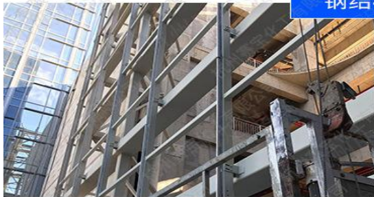
钢结构网架
